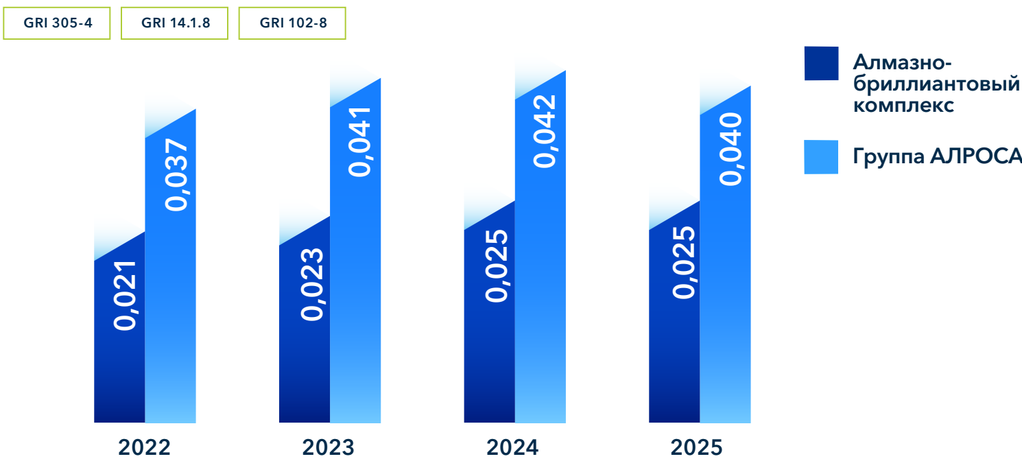
Удельные прямые выбросы парниковых газов (область охвата 1), тонн CO 2 -экв./карат
